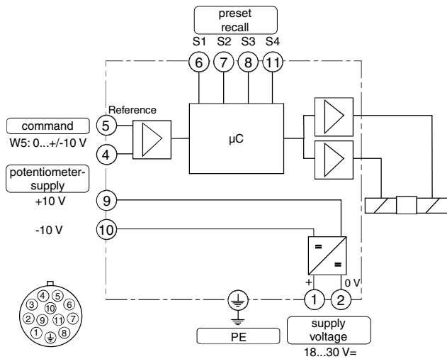
Code W5 11 + PE acc. to EN 175201-804
