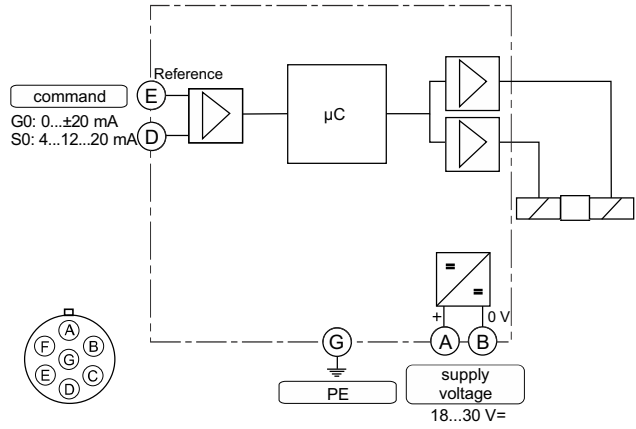
Code G0, S0 6 + PE acc. to EN 175201-804
