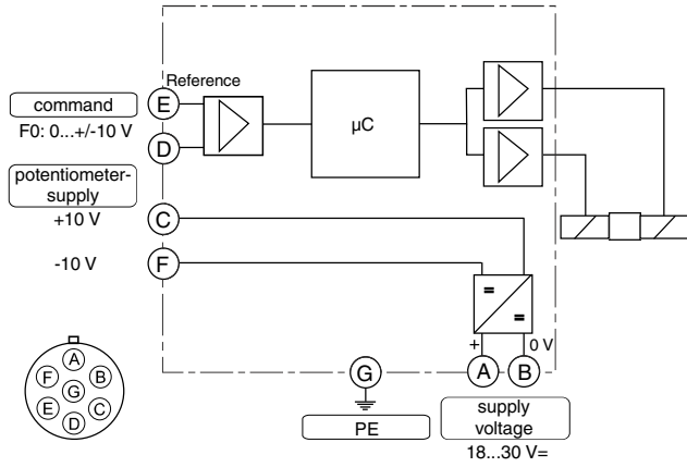
Code F0 6 + PE acc. to EN 175201-804
