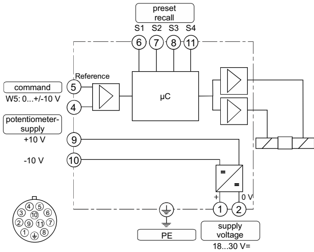
Code W5 11 + PE acc. to EN 175201-804
